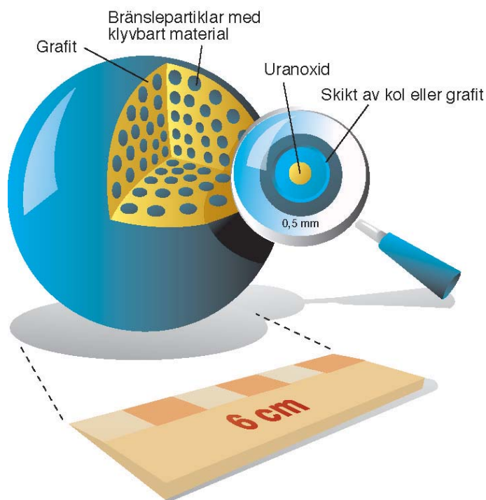
Figur 4. Ny typ av bränsle i pebble-bedreaktorn (PBMR)
